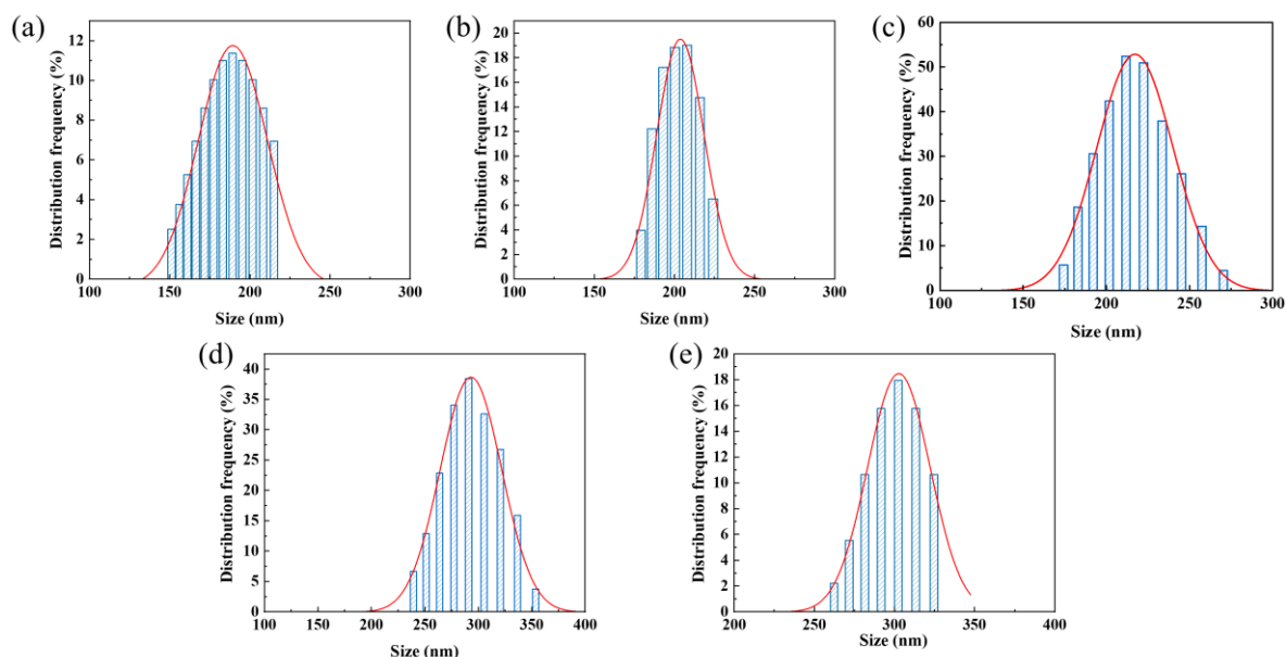
Figure 3: Particle size distributions of representative CNC samples (a) CNC-4, (b) CNC-5, (c) CNC-6, (d) CNC-7, (e) CNC-8
